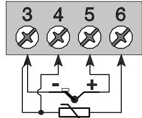
3-хпровод термоэлемент
