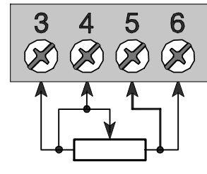
3-хпровод термоэлемент
