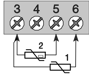
2 ТС, 2-хпроводные
